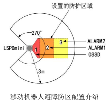
移动机器人避障防区配置介绍
