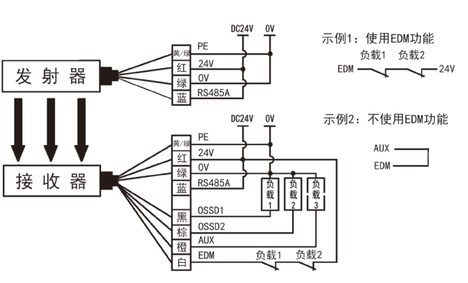
M 型，光同步编码 2 接线图
