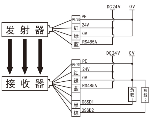
G 型，光同步编码 2 接线图
