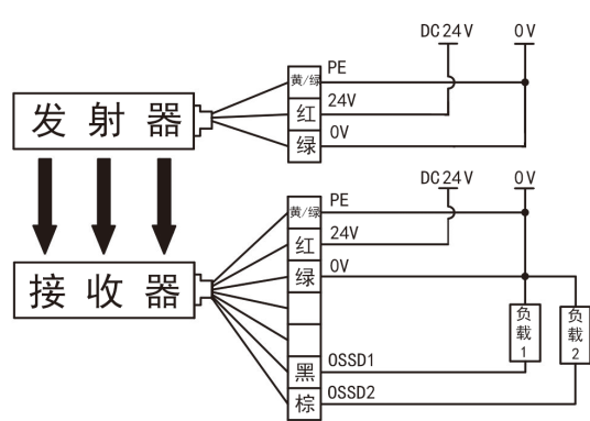
G 型，光同步编码 1 接线图
