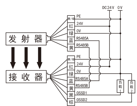
G 型，线同步接线图
