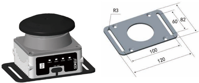
水平安装方式（KLMs-SZ）
