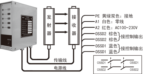
不带附加功能 CG 接线图
