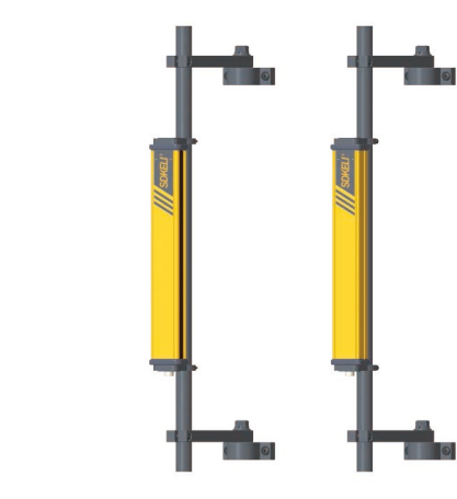
双旋臂支架侧装方式 (G1) 发射器、接收器通过 KS 型管装固定夹固定于钢管支架上, 旋臂座固定在机床底座或立柱上。双旋臂可有效增强抗振性能。
