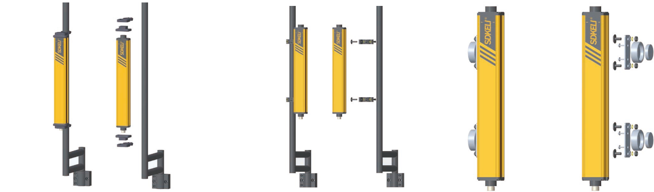
双臂支架侧装 - 带减振器安装方式 (SCJ) 发射器、接收器通过 KS 型管装固定夹固定于双臂管装支架上, 支架座固定在机床底座或立柱上。
