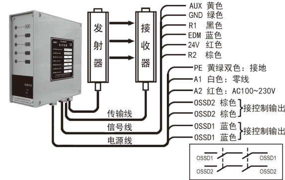
带附加功能的通用继电器型号接线图
