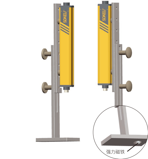
板状支架磁吸安装方式 (BC) 发射器、接收器选用磁吸安装方式安装于板状支架上, 板状支架选用强力磁铁吸于机床作业台面上。采用该安装方式, 必须有专门的安全管理人员负责管理。
