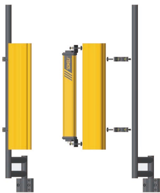
双臂支架配防护罩方式 (SF)
