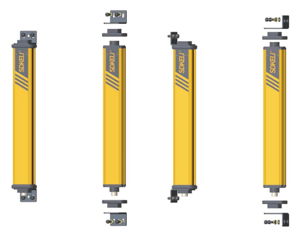
正侧装一体安装方式 (ZC) 将 KS06/KS06G 型发射器、接收器通过 KS 型正侧装支架直接安装于机床床身上的安装方式。
