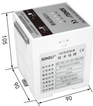
CQ2/CQ5 型控制器
