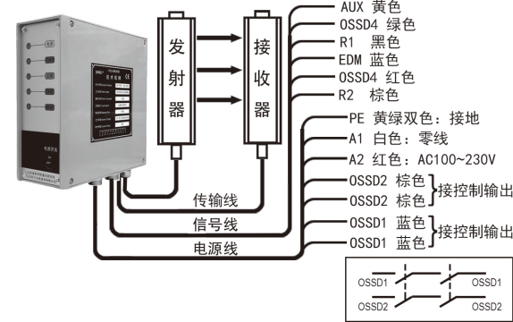
带附加功能的强制导向继电器型号接线图
