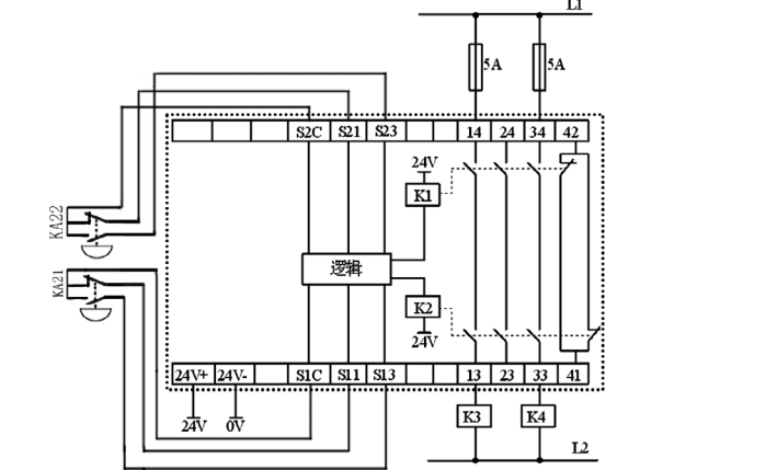
图 13 3A1B 监控双手按钮信号
