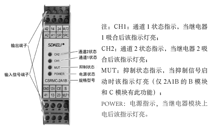
图 16 CSRM 型安全继电器模块面板示例
