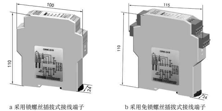
图 15 CSRM 型安全继电器模块外形尺寸图
