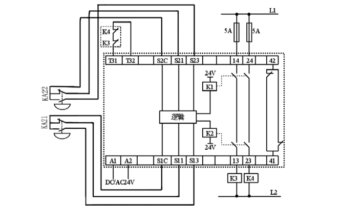
图 13 3A1B 监控双手按钮信号
