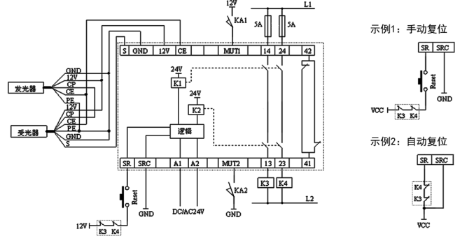
图 11 3A1B 监控光幕信号
