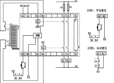
图 2 3A1B 监控急停信号
