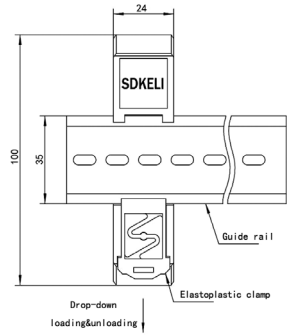
图 17 CSRM 型安全继电器模块安装示意图
