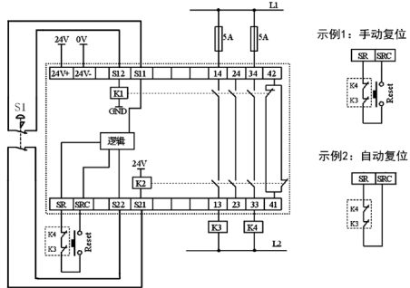
图 2 3A1B 监控急停信号
