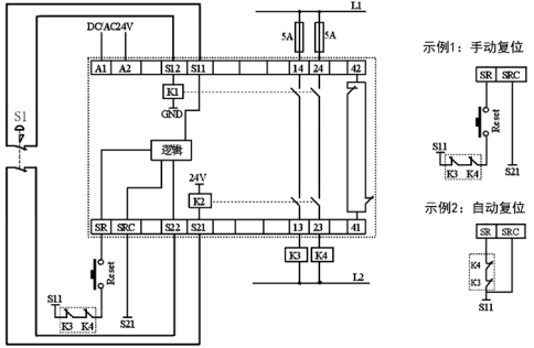
图 3 2A1B 监控安全门信号
