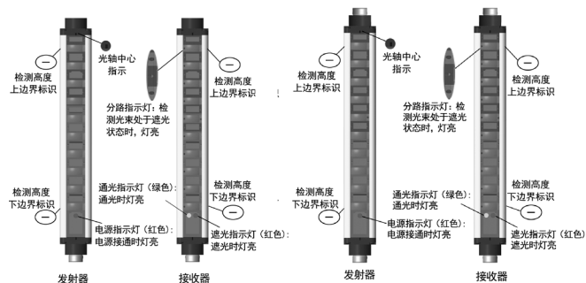
图 1.1.1 主光栅
