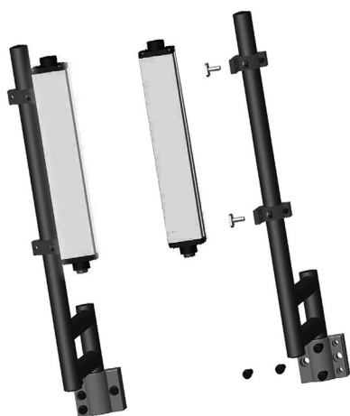
7.4 双臂支架侧装-T型槽安装方式 (SCT)
