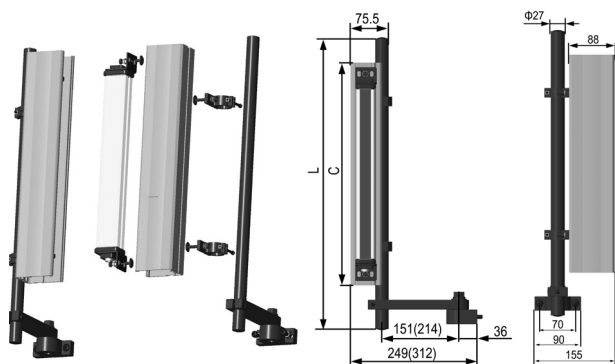
7.8 管装支架配防护罩 (GF)
