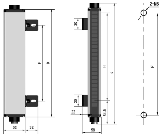
7.6 防护罩正装方式 (FZ)
