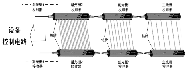
图 7 KS06G 型级连式安全光栅连接示意图
