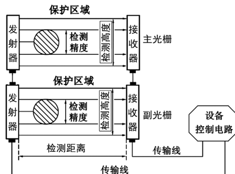
图 1 级连式安全光栅工作示意图
