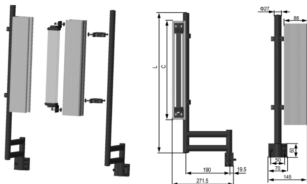
7.9 双臂支架配防护罩方式 (SF)
