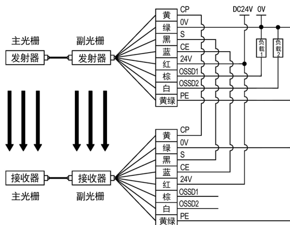
8.2、NPN 输出型接线图
