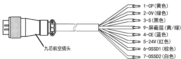
图 1.2.2 KS06G 型级连式安全光栅单端传输线
