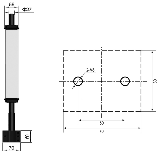
7.4 双臂支架侧装-T型槽安装方式 (SCT)
