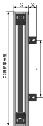
7.7 防护罩侧装方式 (FC)
