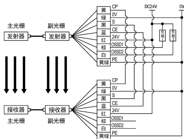
8.2、NPN 输出型接线图
