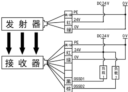
(2) NPN，光同步，光通信编码 2
