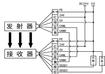
(3) PNP，线同步
