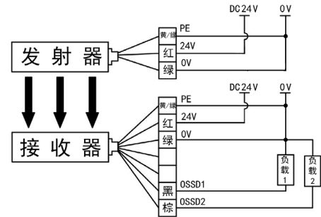
(2) PNP，光同步，光通信编码 2
