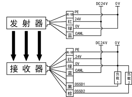
(2) PNP，光同步，光通信编码 2
