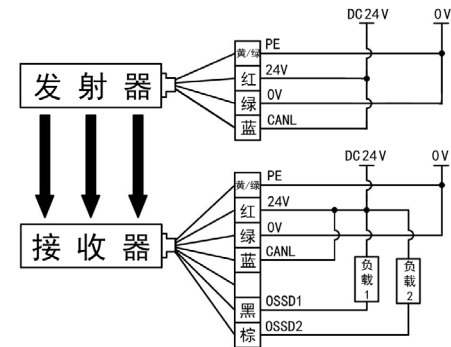
(3) NPN，线同步
