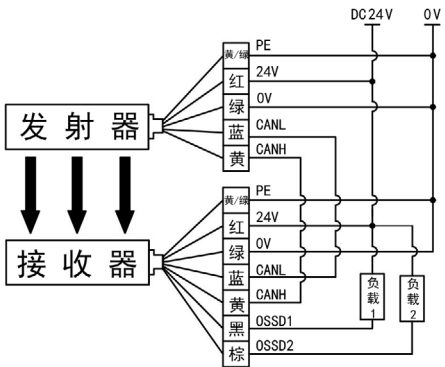
(3) NPN，线同步
